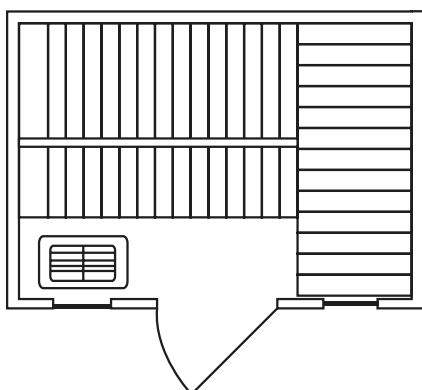
9806-520 PS57 Sauna para 4 personas con calentador de 6.0 KW de 1.52m x 2.13m
